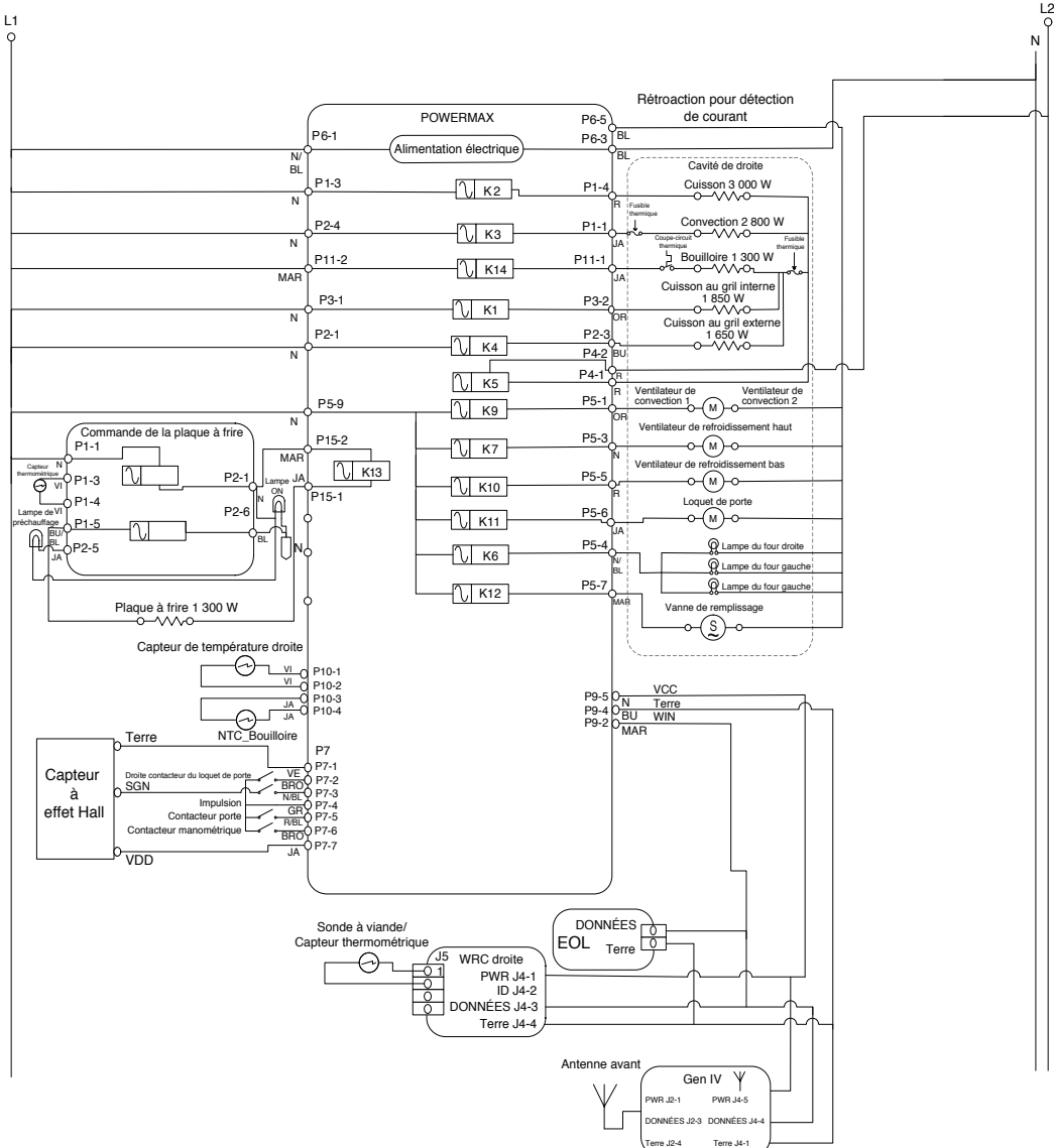
SCHÉMA DE CÂBLAGE Schéma de câblage du module de commande du four
